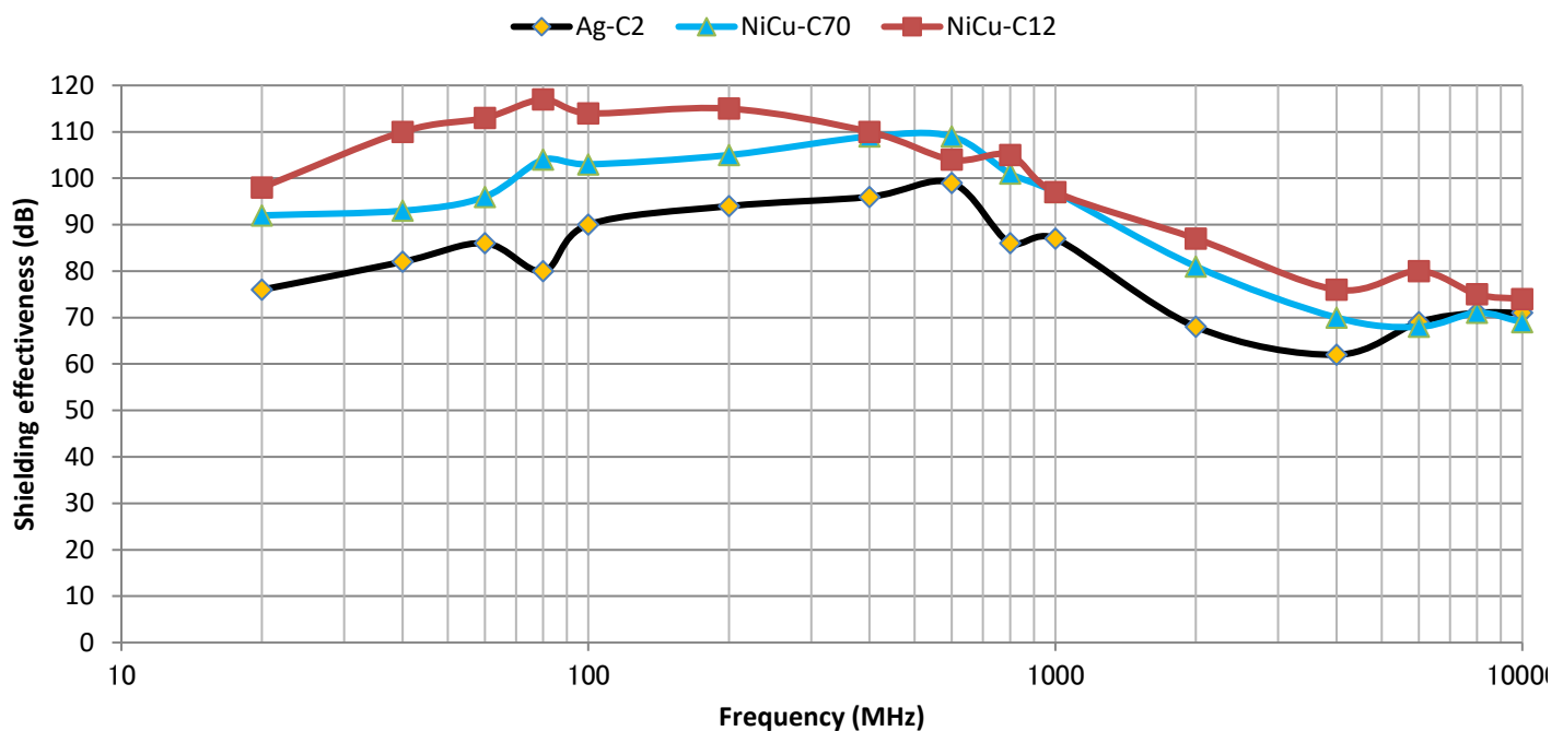
MIL DTL 83528 C シールド効果
